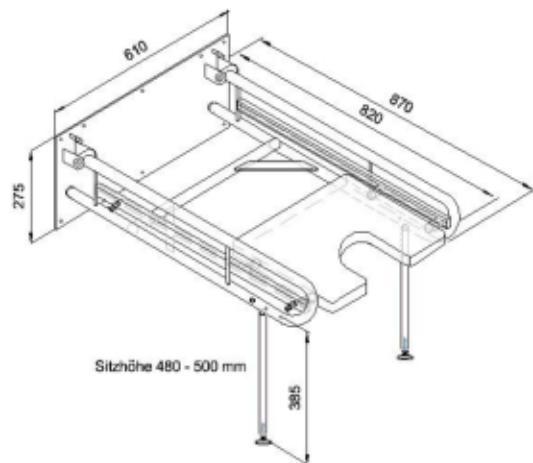
technische Zeichnung
